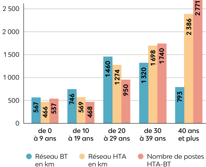
› Ouvrages par tranches d'âge, en 2022
