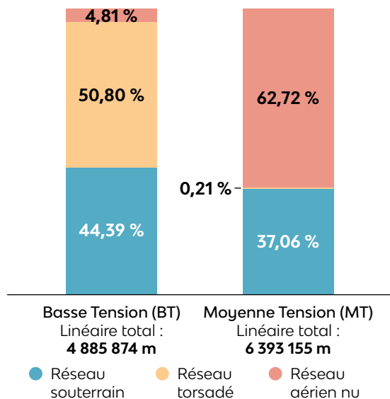
› Répartition par type de réseau, en 2022
